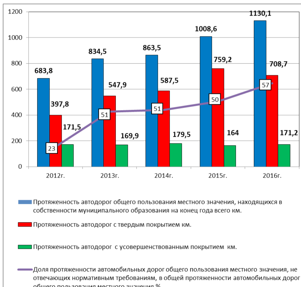
Рис. Протяженность автодорог общего пользования, км.
